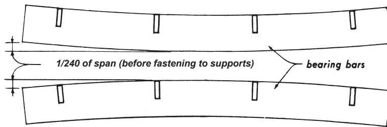
longitudinal bow
